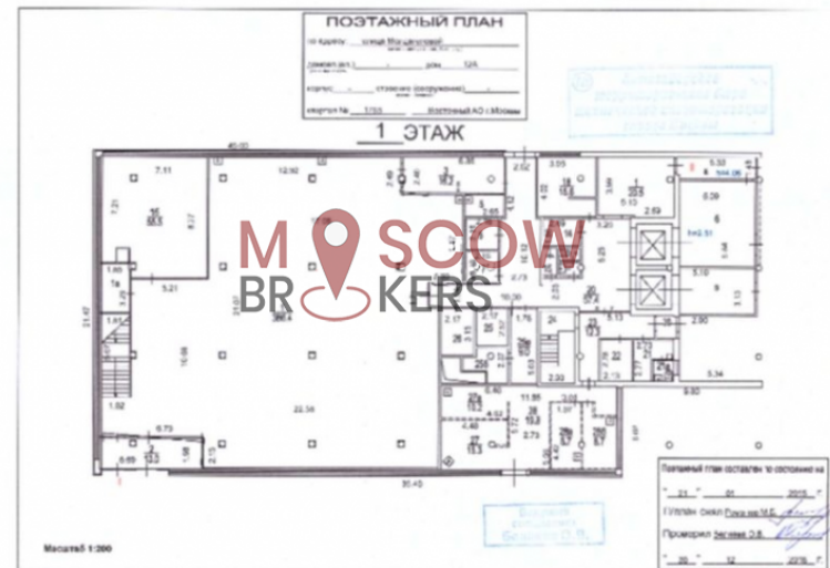
Поэтажный план. 1 этаж
