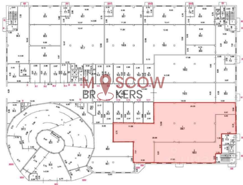
1-й этаж
